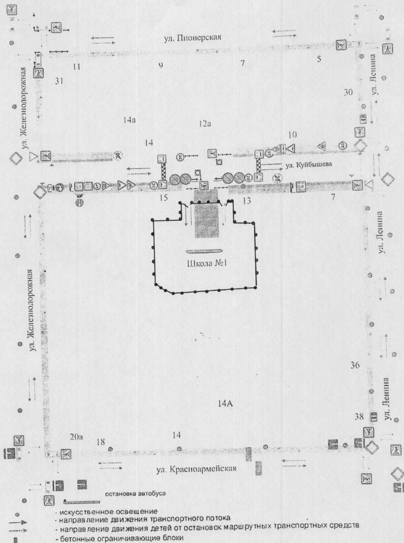
Схема безопасного расположения остановки автобуса у образовательной организации
